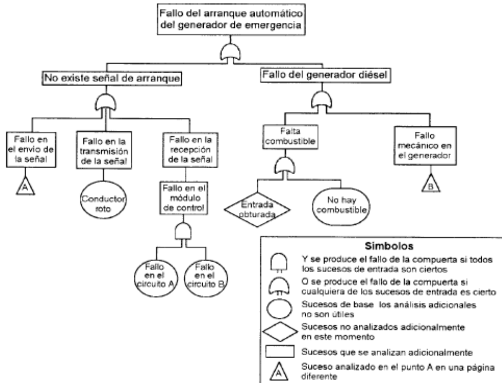
Figura B.2 - Ejemplo de un FTA según la Norma IEC 60300-3-9
