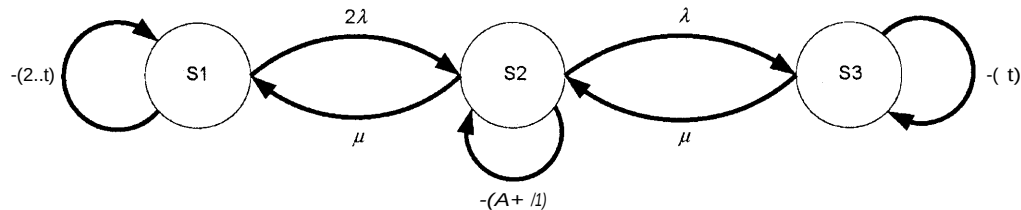
Figura B.10- Ejemplo de diagrama de transición de estado
