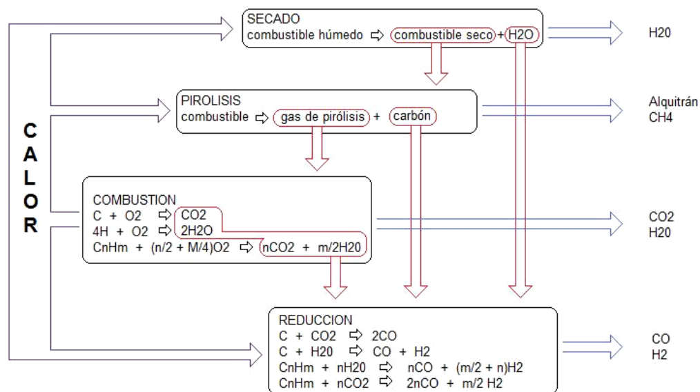
Figura 1.6 Etapas de la gasificación.
