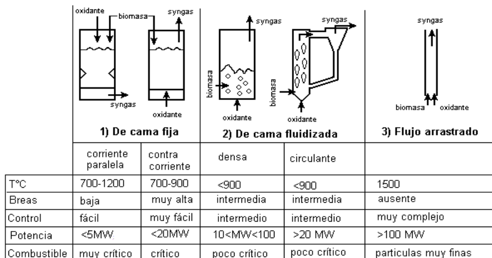
Figura 1.7 Cuadro comparativo entre los distintos tipos de gasificadores.
