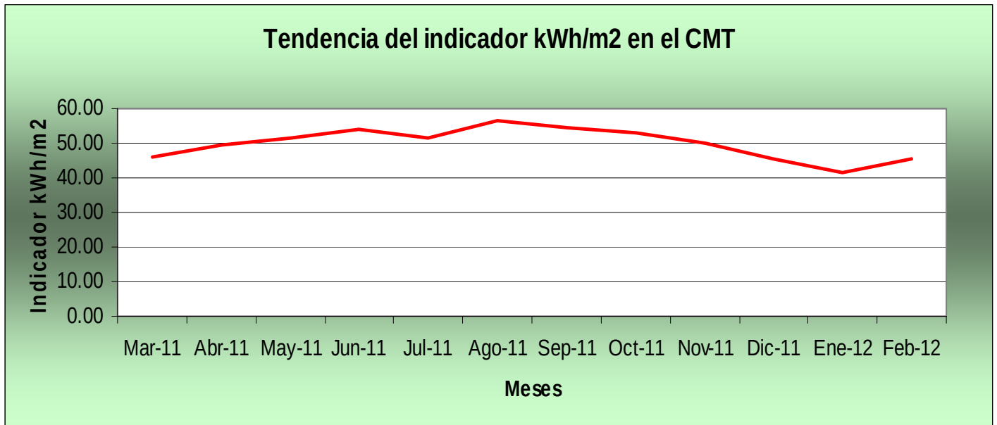
Figura 3.3. Comportamiento del indicador kWh/m 2 en el local del CMT.
