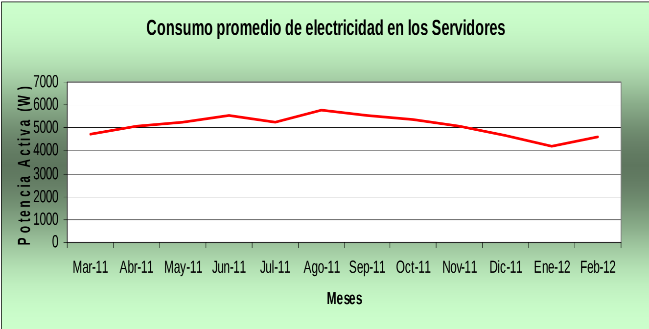
Figura 3.2. Comportamiento del consumo promedio de electricidad en el local Servidores en los doce meses.
