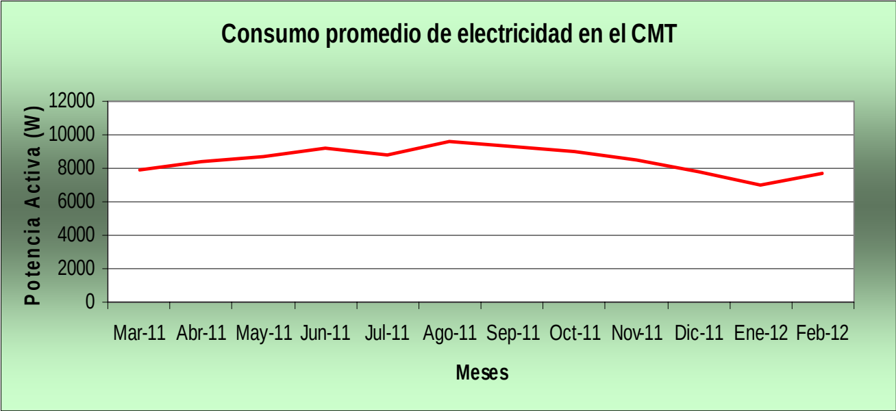
Figura 3.1. Comportamiento del consumo promedio de electricidad en el local CMT en los doce meses.
