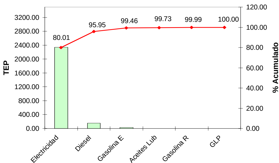
Figura 2.2 Estructura de consumo en toneladas de combustible convencional (TCC) de los portadores energéticos en el año 2011.
