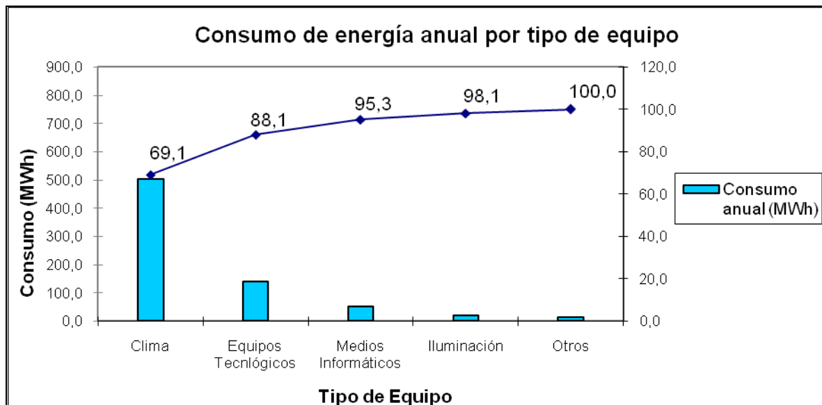
Figura 2.3 Estratificación del edificio de la Dirección Territorial por tipo de equipos.
