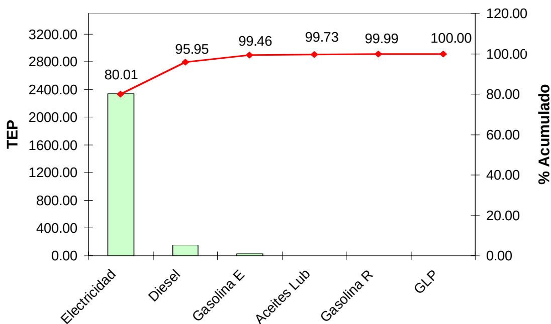
Figura 1.5 Estructura de consumo en toneladas de combustible convencional (TCC) de los portadores energéticos en el año 2011.
