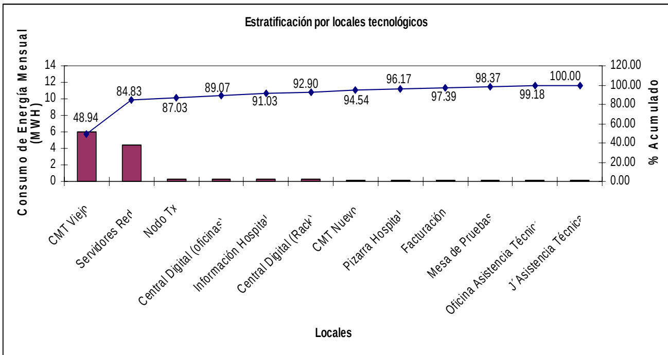
Figura 2.5. Estratificación del Clima Tecnológico en el Edificio de la Dirección Territorial.
