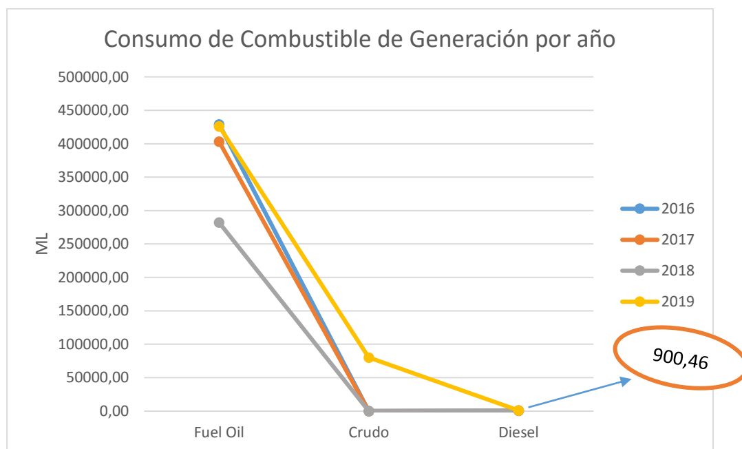
Figura 3.4: Consumo de Combustible de Generación por año. Fuente: Elaboración Propia.
