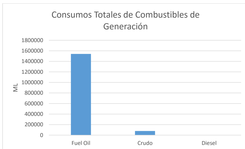
Figura 3.5: Consumos Totales de combustibles en los 4 años estudiados. Fuente: Elaboración Propia.
