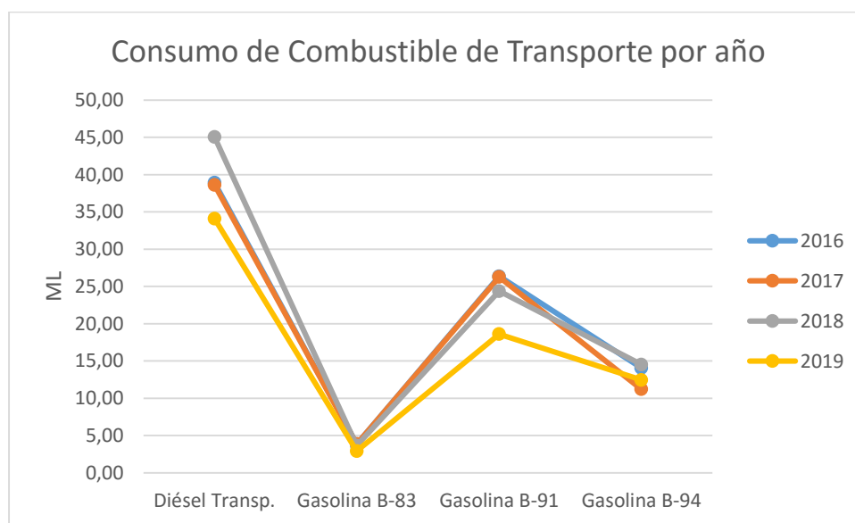
Figura 3.6: Consumo de combustible por años. Fuente: Elaboración Propia.
