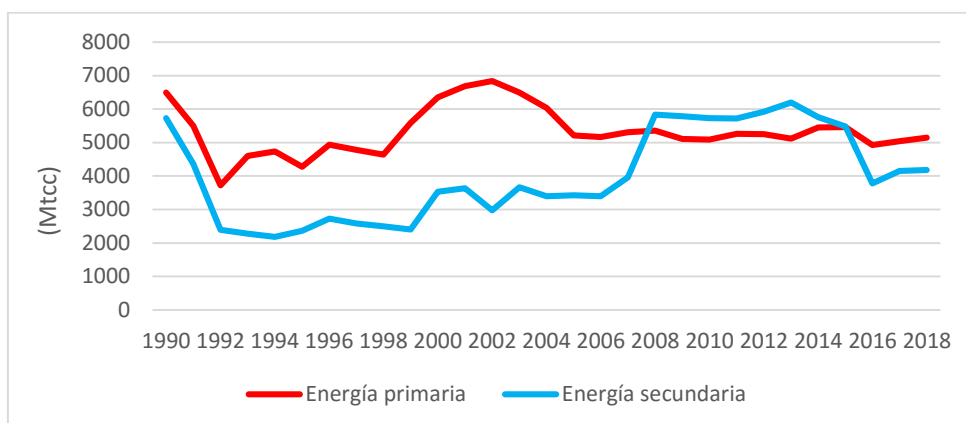
Figura 2.2: Producción de energía primaria y secundaria en Cuba. Fuente: (Campillo Sabina, 2018).
