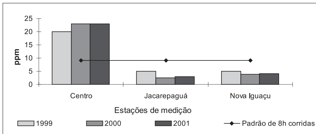
Figura 4.14 Concentração média de oito horas corridas de monóxido de carbono (CO)
