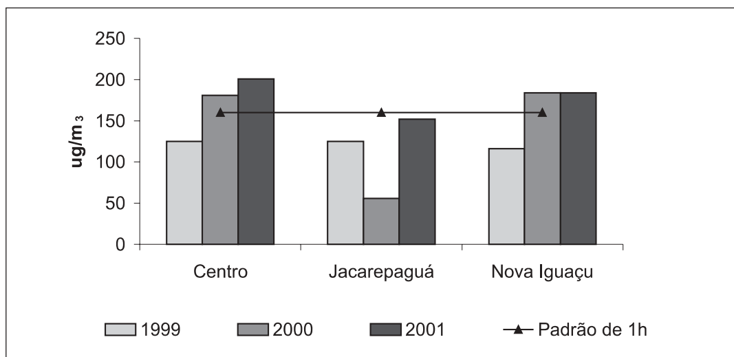
Figura 4.16 Concentração máxima horária de ozônio ( O_3 )
