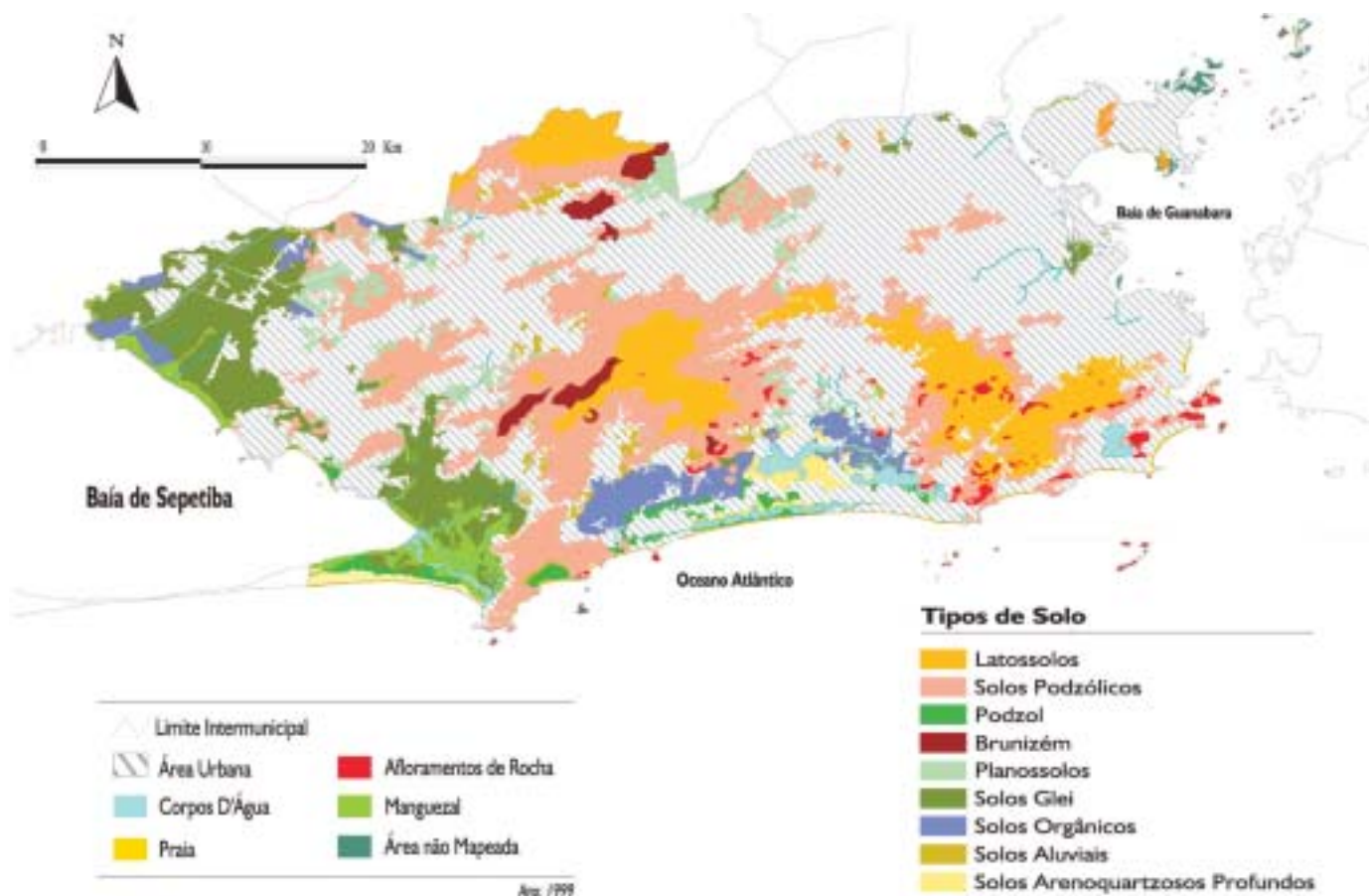
Figura 4.5 Semidetalhamento dos Solos
