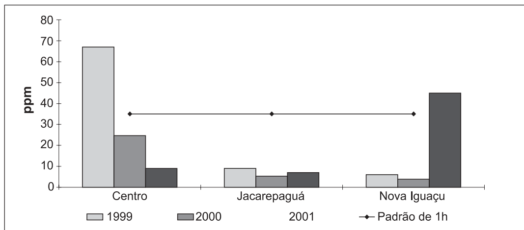
Figura 4.15 Concentração máxima de 1 hora de monóxido de carbono (CO)
