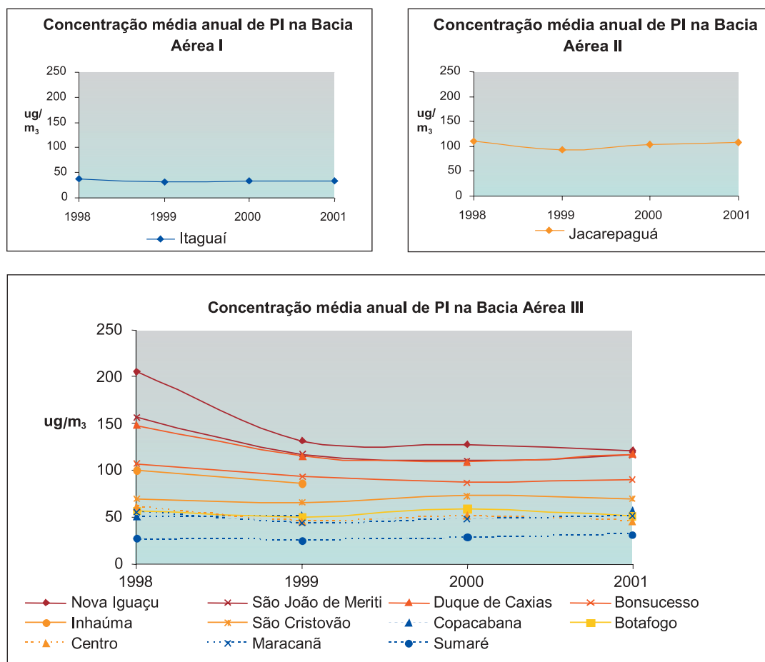
Figura 4.10 Concentrações médias anuais de partículas inaláveis (PI).
