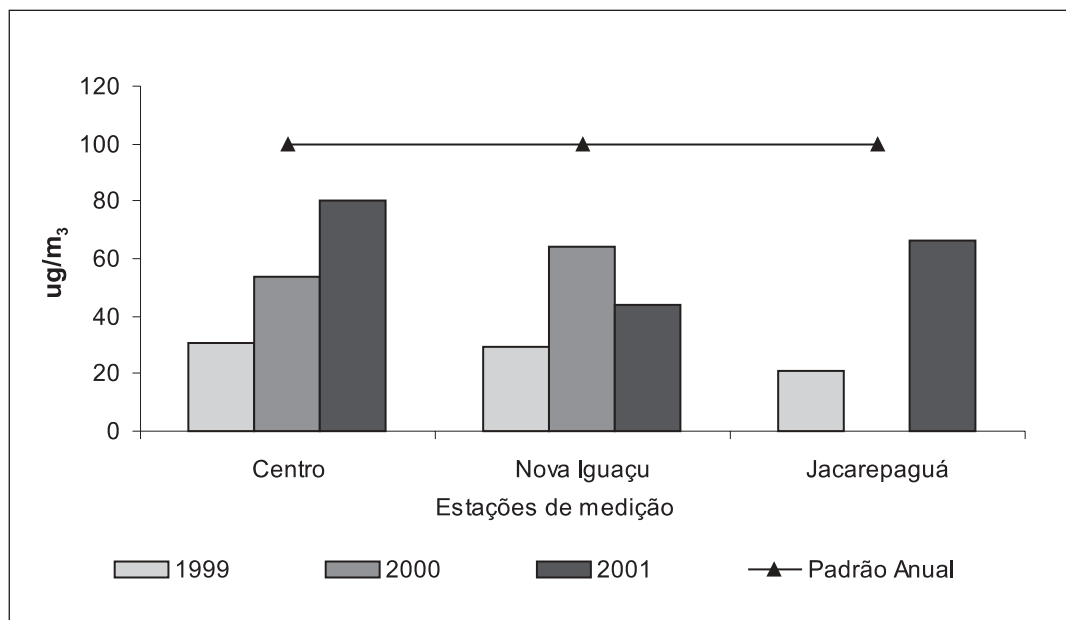
Figura 4.13 Concentração média anual de dióxido de nitrogênio ( \text{NO}_2 )
