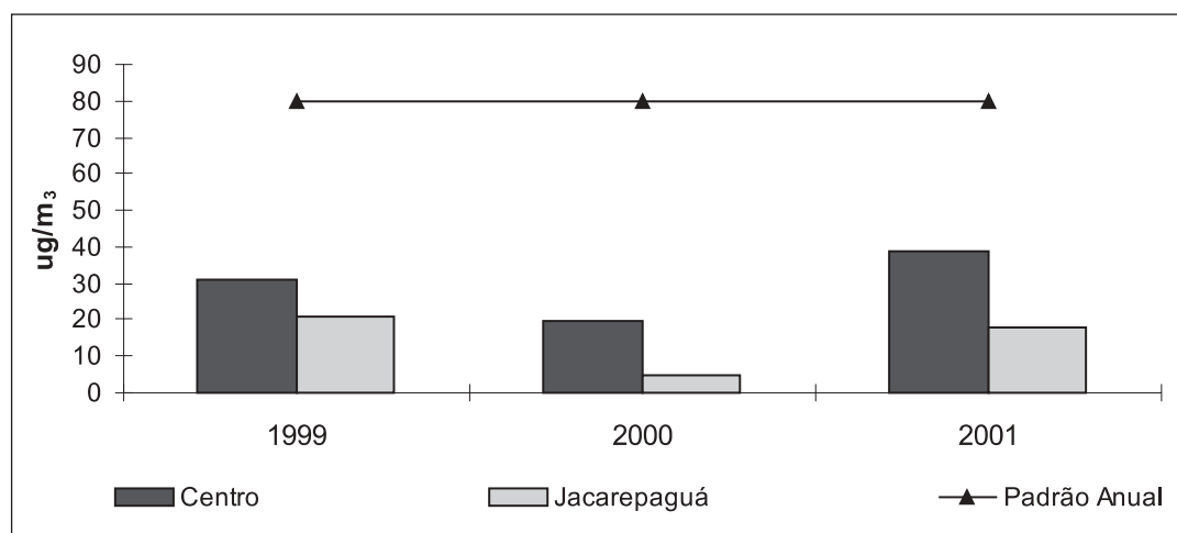
Figura 4.12 Concentração média anual de dióxido de enxofre ( \text{SO}_2 )
