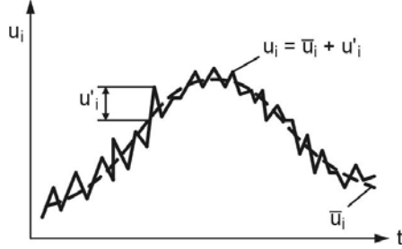
Fig. 3.9. Unsteady turbulent flow
