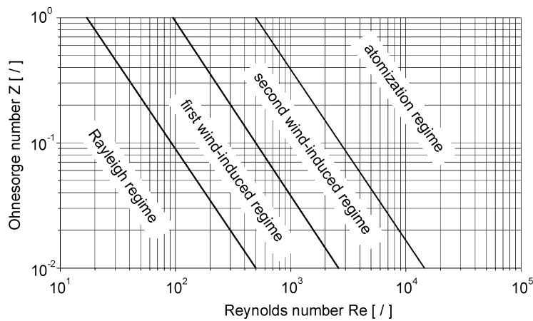
Fig. 2.1. Ohnesorge diagram: jet break-up regimes
