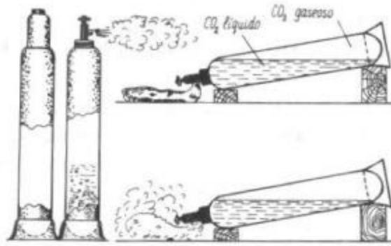
Figura 98. A la izquierda: anhídrido carbónico contenido en una botella de acero de paredes gruesas; encima están sus vapores. Más a la derecha: cuando se abre la válvula el líquido comienza a bullir a consecuencia del descenso de presión. A la derecha arriba: la botella está inclinada para verter anhídrido carbónico en un saco atado al grifo. A la derecha abajo: el saco queda envuelto en una nube de vapores de anhídrido carbónico condensados; dentro del mismo se encuentra anhídrido carbónico congelado.
