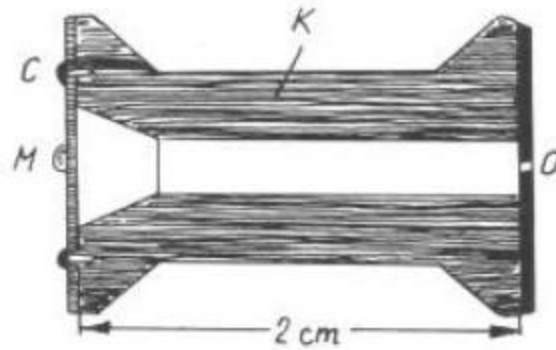
Figura 106. La Luna vista en un carrito de madera. El objeto se pega a un círculo de celuloide transparente C y se examina a través de un diminuto orificio O, practicado en el círculo de cartulina P. El interior del carrito está pintado de negro.
