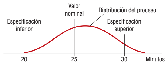
(b) El proceso no es capaz
