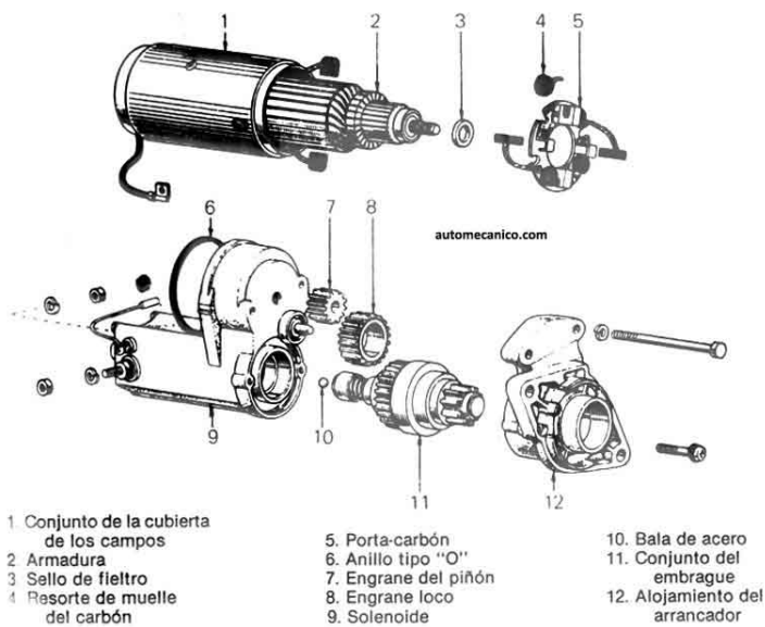
Vista esquemática de la reducción de engranes del motor de arranque.
