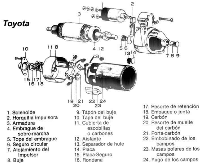
Vista esquemática del motor de arranque.
