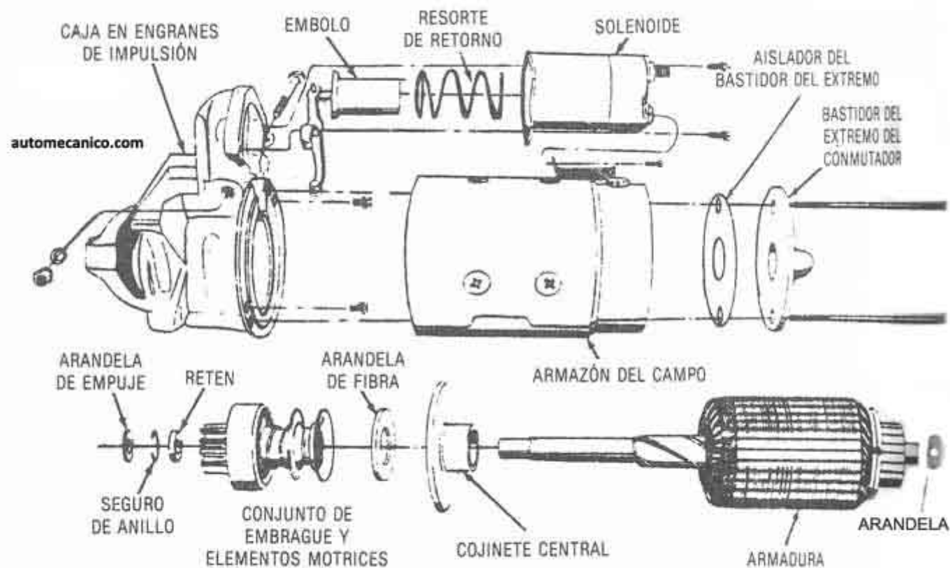
General Motors 350 V8 diesel, vista de despiece del motor de arranque (© Div. OLDSMOBILE G.M. Corp.).
