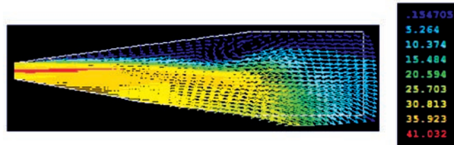
FIGURA 6. Gráfico de modelación de la corriente de aire del pulverizador SS800 moviéndose a una velocidad de 2,18 km/h.
