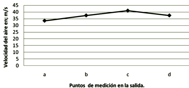
FIGURA 4. Distribución de velocidad del aire a la salida del ventilador utilizado en la modelación.
