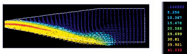
FIGURA 7. Gráfico de modelación de la corriente de aire del pulverizador SS800 moviéndose a una velocidad de 4,5 km/h.
