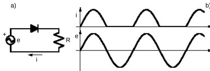
Fig. 1.- La curva superior de 1b) representa la intensidad por el alternador de la figura 1a). No es alterna, sino rectificadora de media onda.
