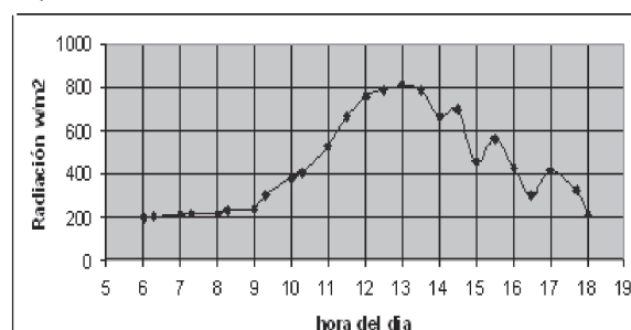
Figura 7. Comportamiento de la radiación solar típica del trópico
