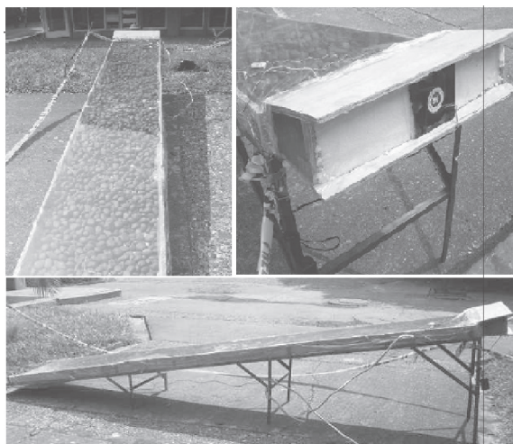
Figura 13. Colector solar de lecho de rocas
