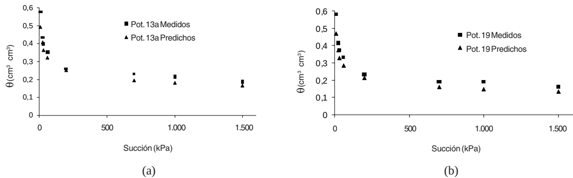
Figura 3. Valores de contenido de humedad medidos y predichos por las FPT de Saxton y Rawls, en función del potencial mátrico para el Potrero 13a (a) y el Potrero 19 (b). Figure 3. Measured and predicted soil water content values from FPT of Saxton and Rawls, as a function of matric potential for 13a (a) and 19 (b) plots.
